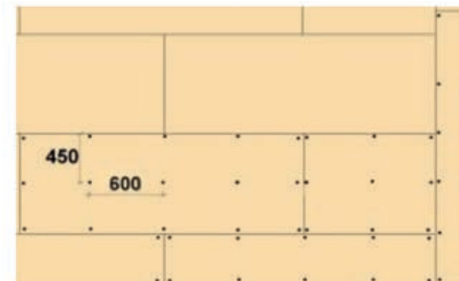
Vaihe 9.
