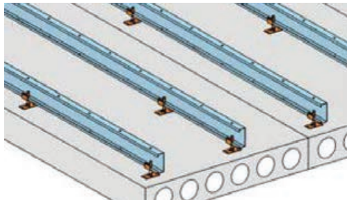
Vaihe 3.
