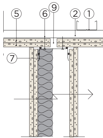
B Pystyleikkaus
