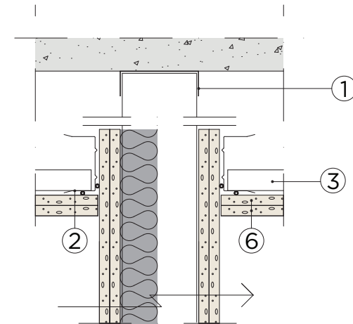
B Pystyleikkaus
