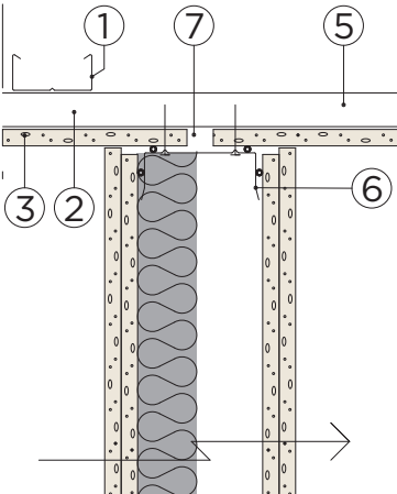
A Pystyleikkaus
