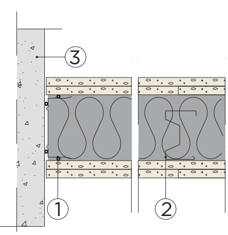
A Vaakaleikkaus
