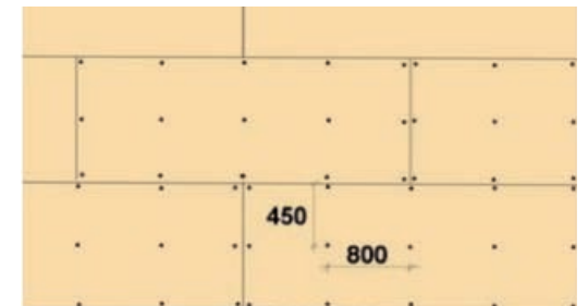
Vaihe 11.
