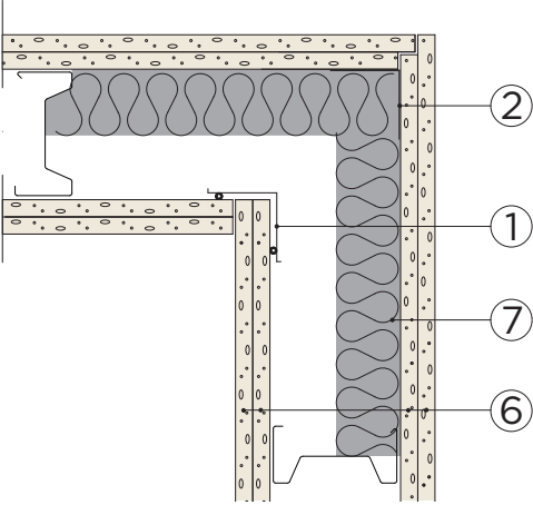
A Vaakaleikkaus
