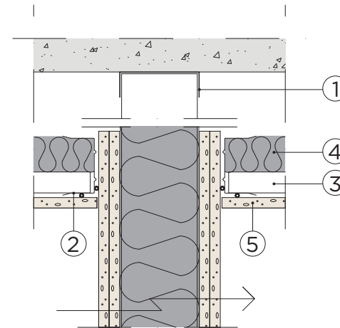
A Pystyleikkaus
