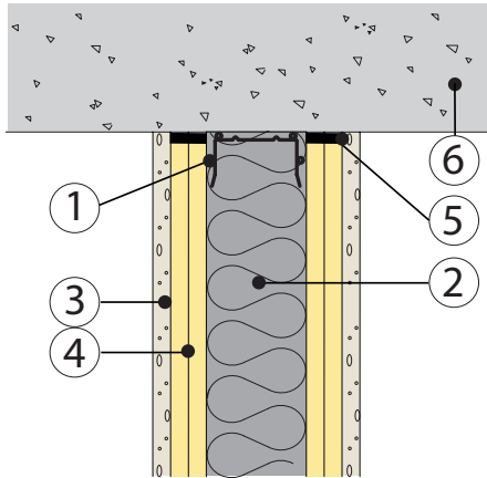
Pystyleikkaus
