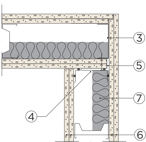
B Vaakaleikkaus
