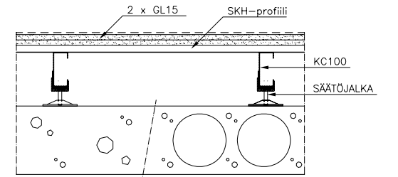
Perusrakenne
