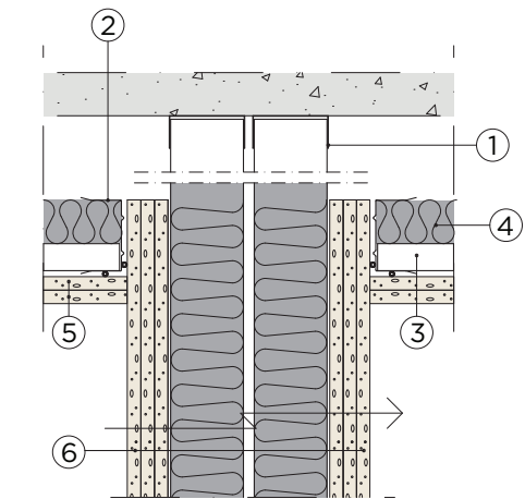
B Pystyleikkaus
