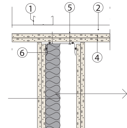
B Pystyleikkaus
