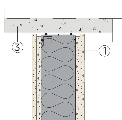
B Pystyleikkaus
