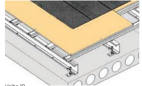
Vaihe 10.
