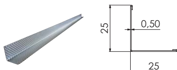
L-lista Glasroc F Palonsuojalevyjen kiinnittämiseen taustarakenteeseen.
