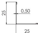
L-lista Glasroc F Palonsuojalevyjen kiinnittämiseen taustarakenteeseen.
